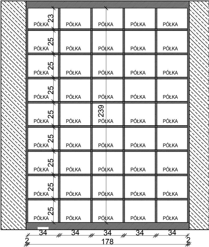
WIDOK ŚRODKA
