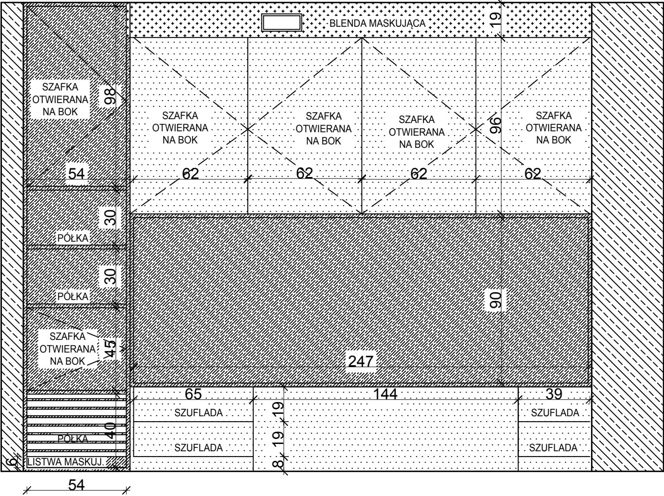
WIDOK FRONTU
