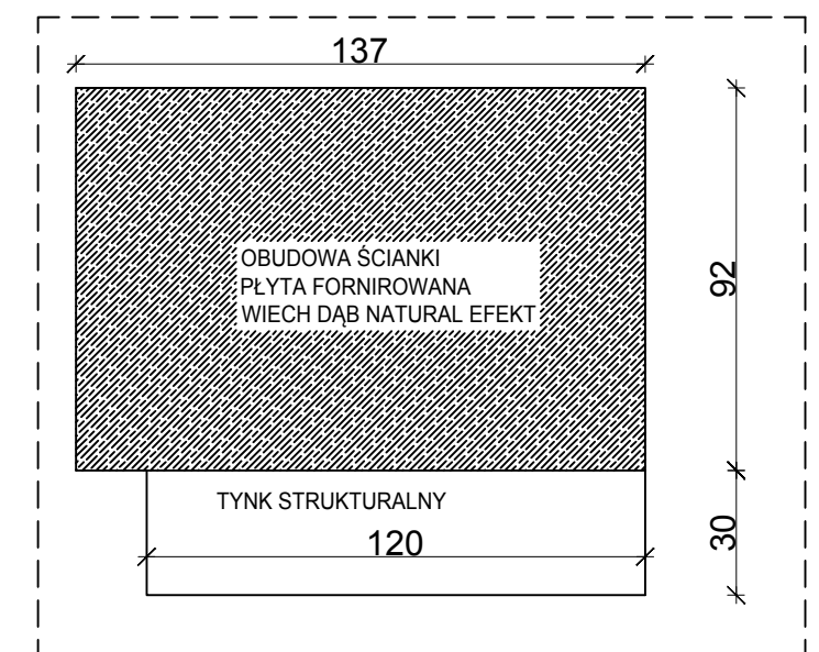
DETAL A WIDOK 2
