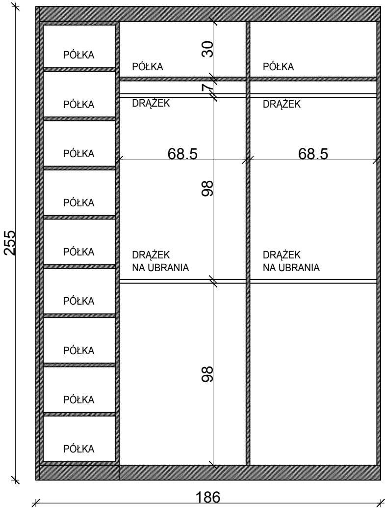
WIDOK ŚRODKA
