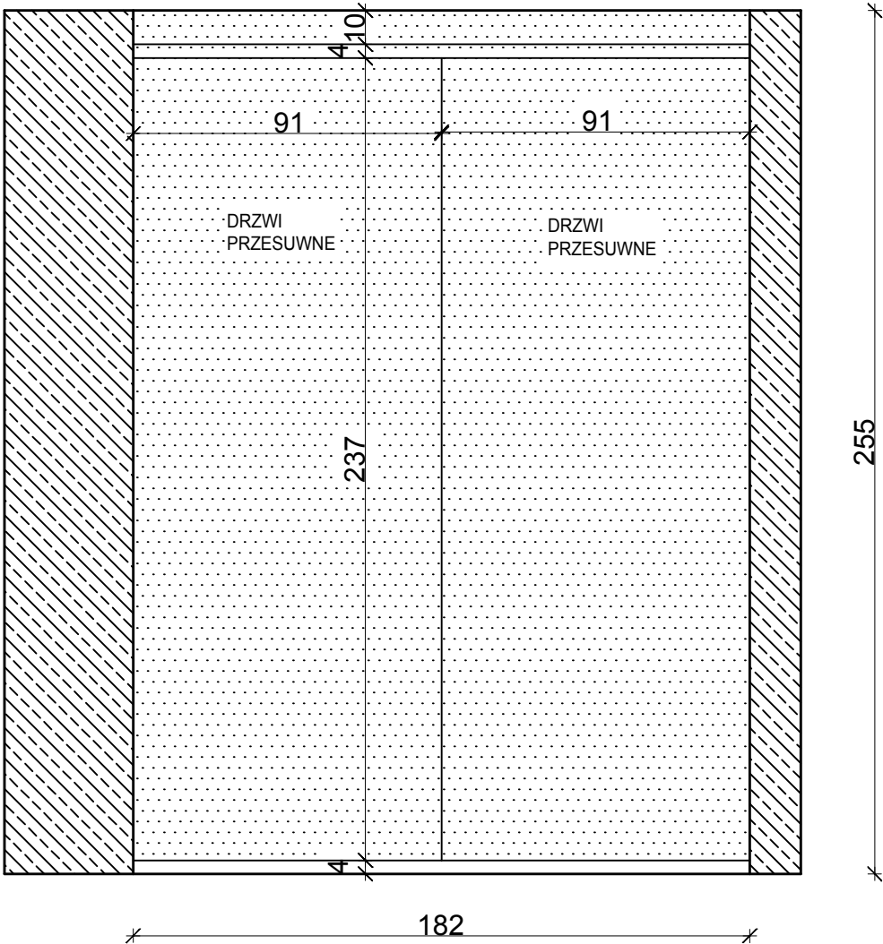
WIDOK FRONTU
