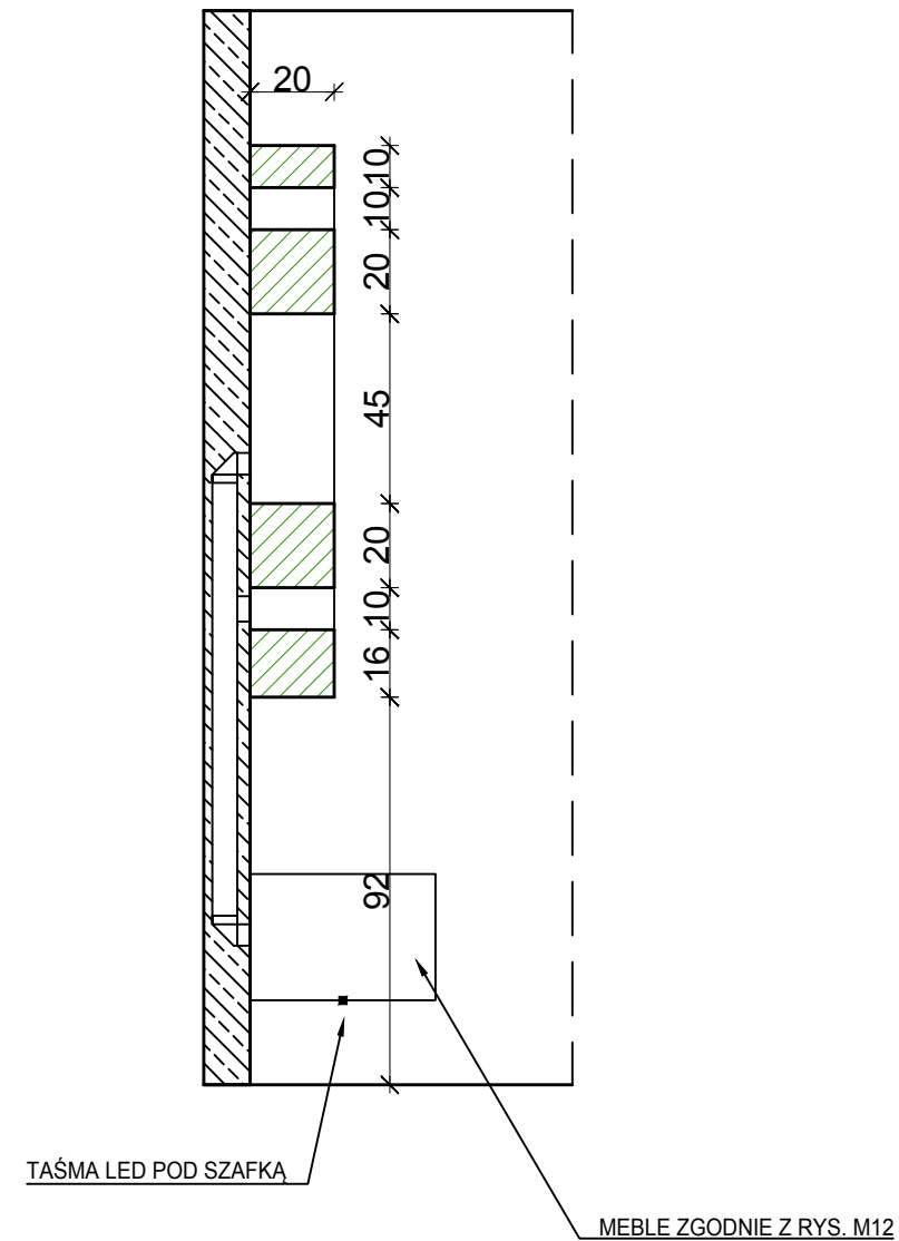
PRZEKRÓJ A-A
