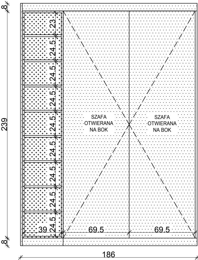
WIDOK FRONTU
