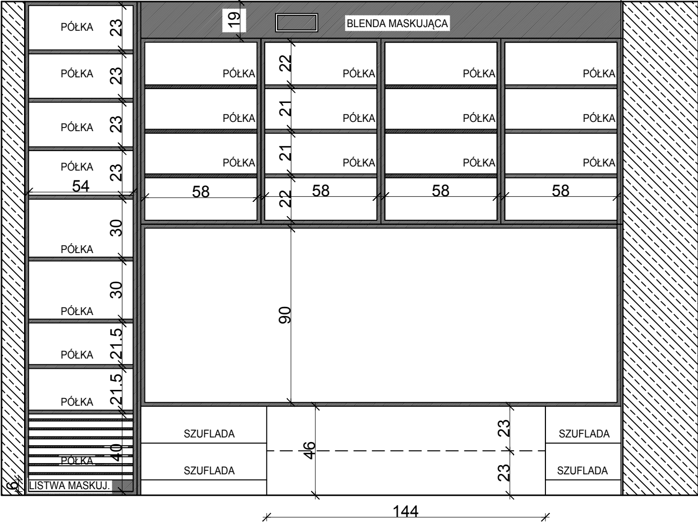
ELEMENT B I C - ZABUDOWA WOKÓŁ ŁÓŻKA
