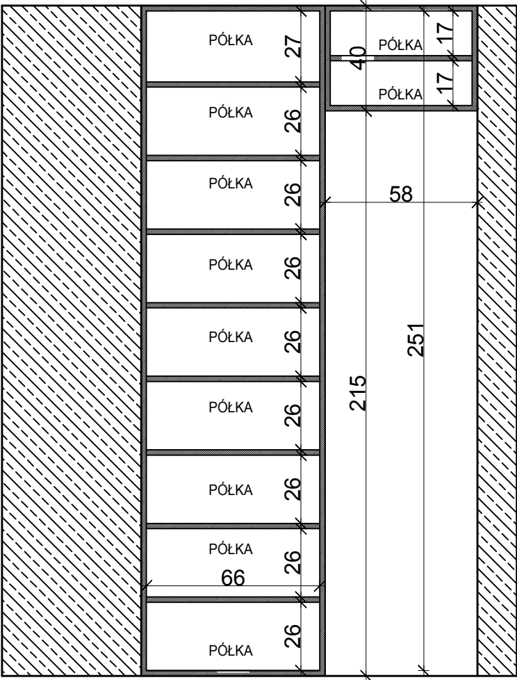
WIDOK FRONTU I ŚRODKA SZAFKI WISZĄCEJ
