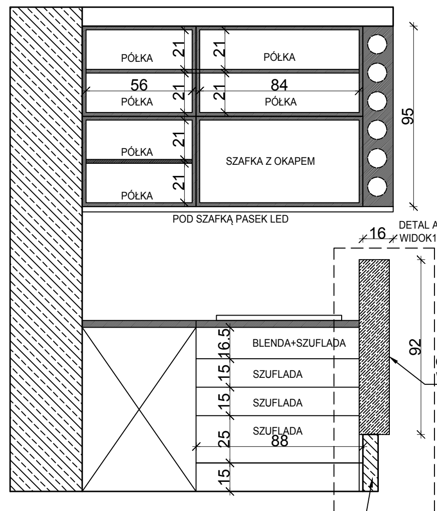
WIDOK WŚRODKU
