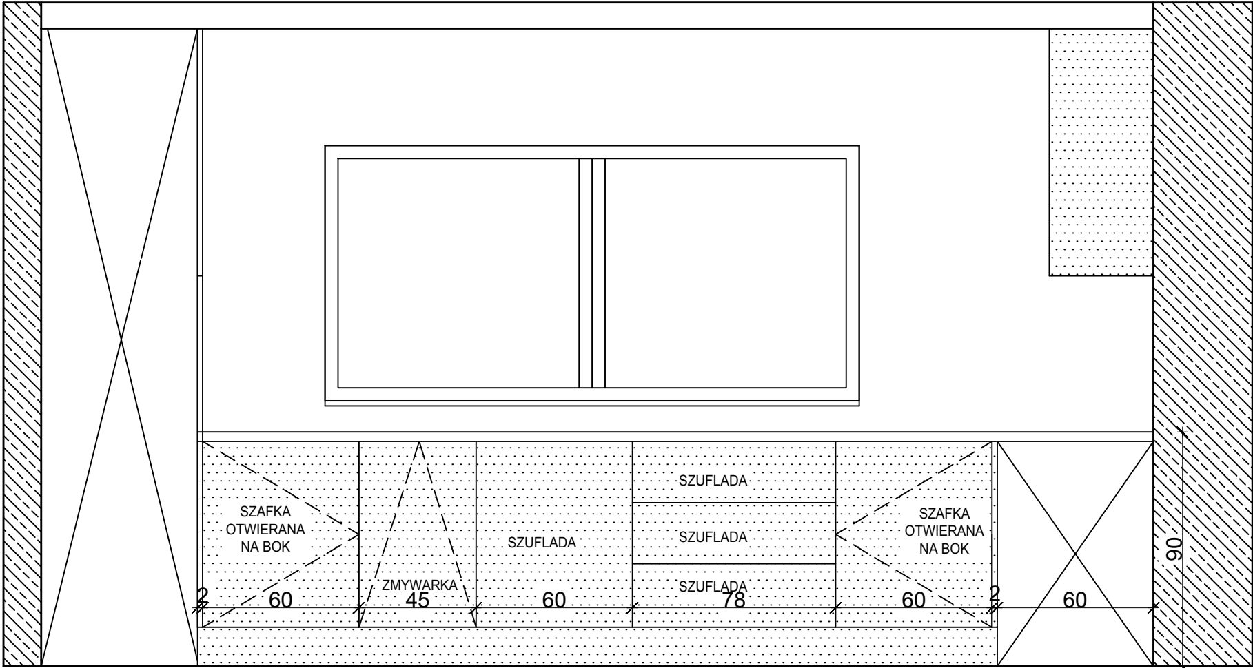
WIDOK FRONTU
