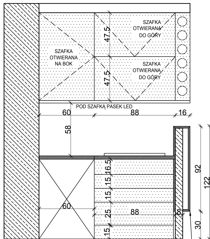
WIDOK FRONTU
