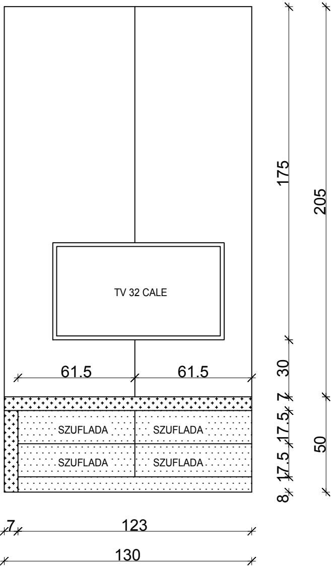
WIDOK FRONTU
