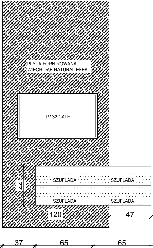
WIDOK FRONTU
