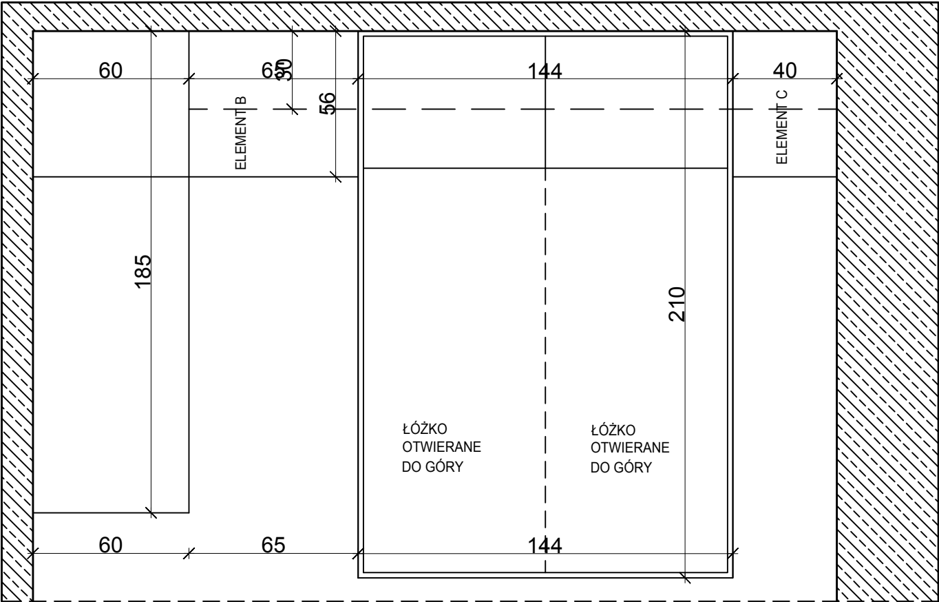
WIDOK FRONTU
