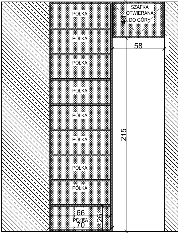
WIDOK FRONTU
