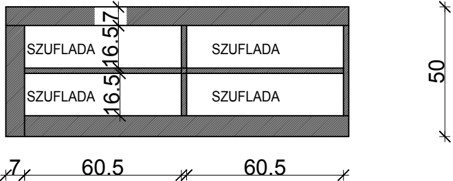
WIDOK ŚRODKA
