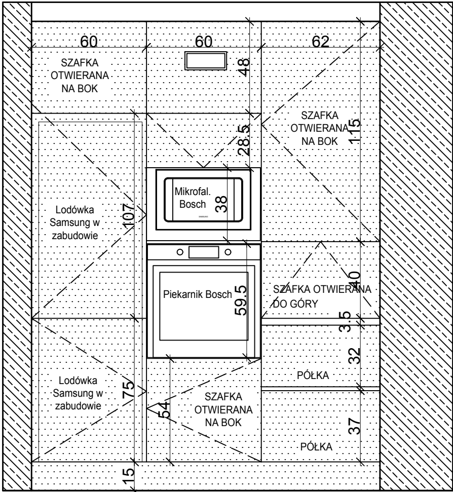
WIDOK FRONTU
